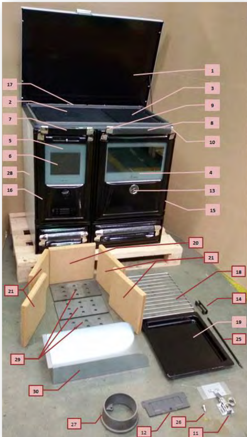
Figura n°25 - Vulcano 7T
