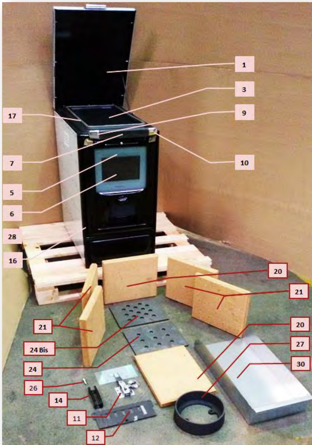
Figura nº24 - Vulcano 4T
