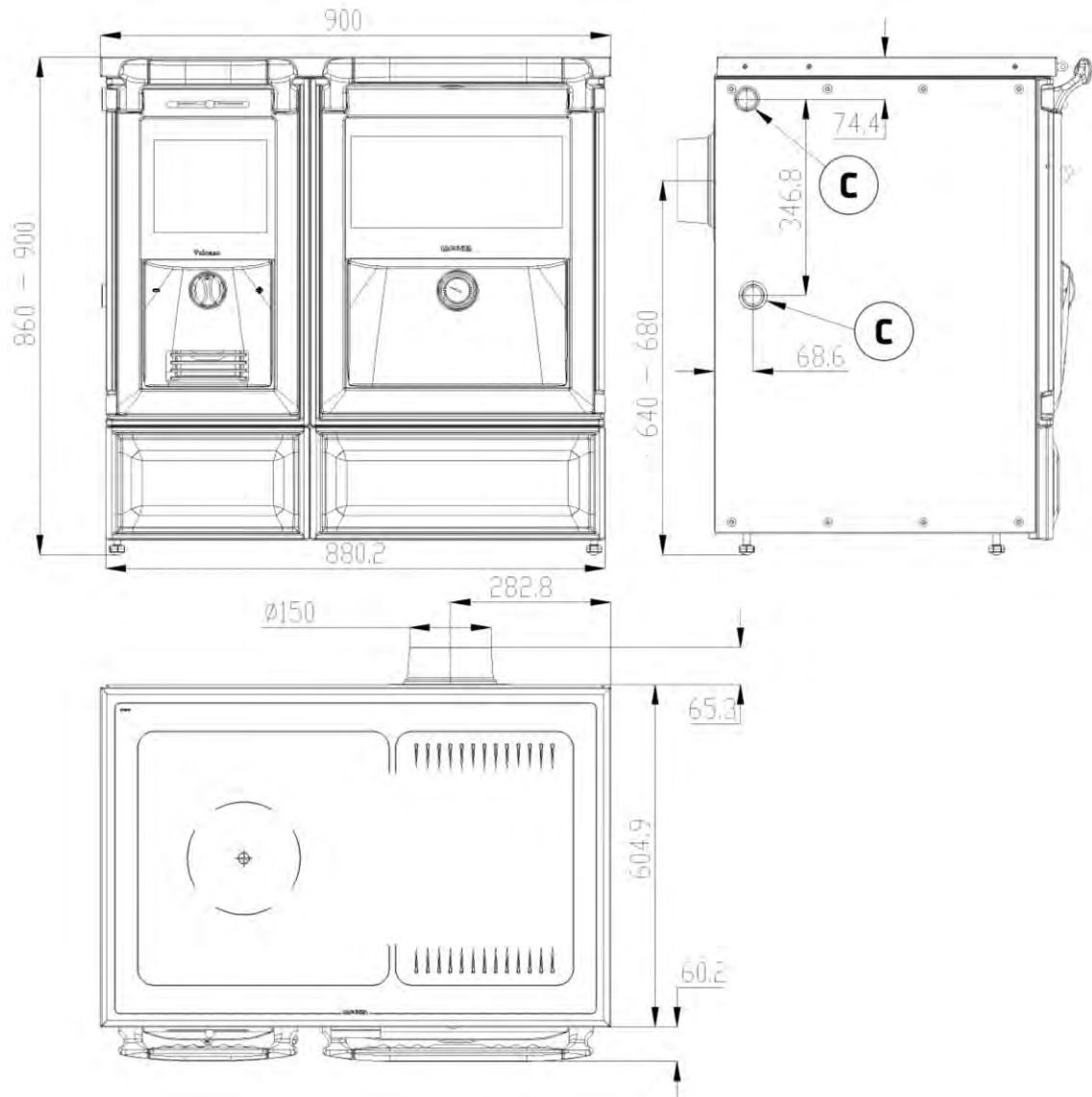
Figura nº2 - Dimensiones en mm del aparato Vulcano 7T E3
