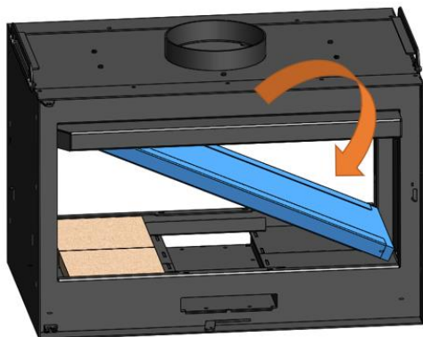
Figura n°18 - Solte o defletor e retire-o da fornalha
