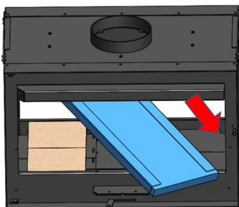
Figura n°19 - Extraia o defletor
