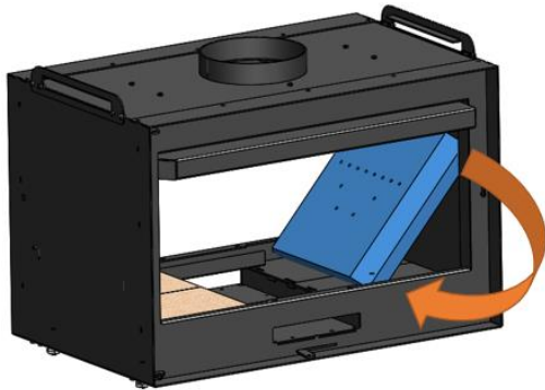
Figura n°17 - Dobramos o refratário lateral para que o defletor caia
