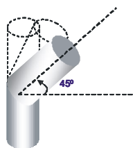
Fig.2–Inclinação correcta para as curvas
