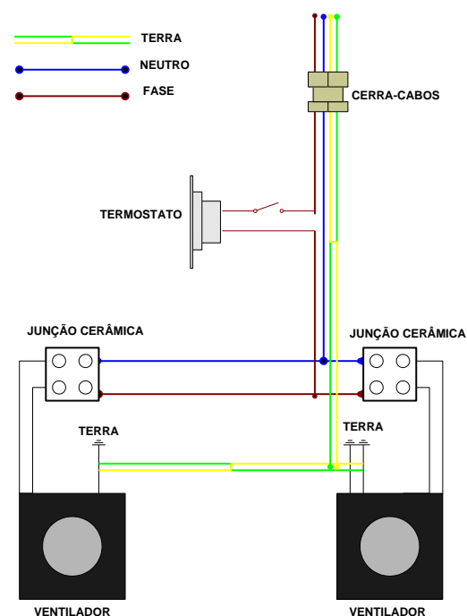
Fig. 4 – Esquema Eléctrico
